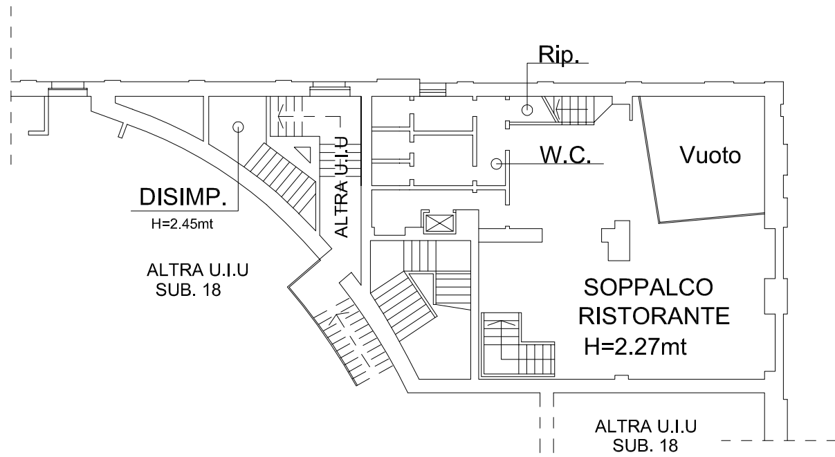
PIANTA PIANO AMMEZZATO
